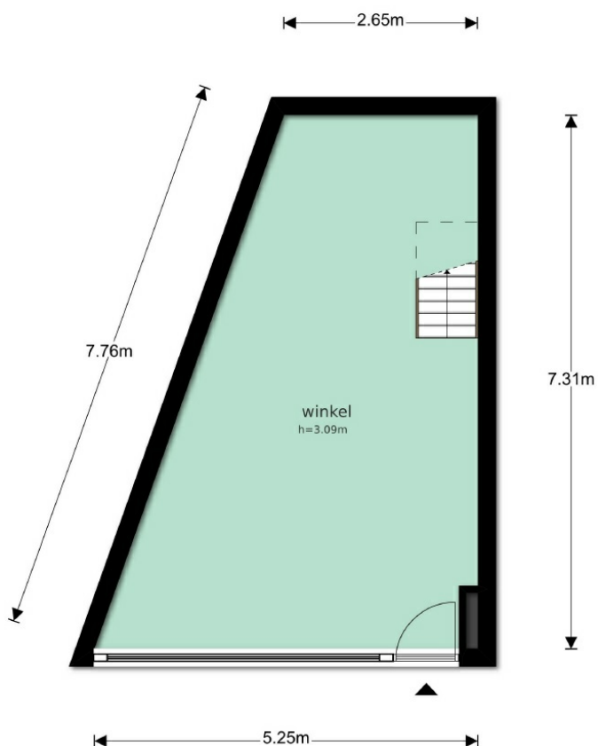
Begane Grond
