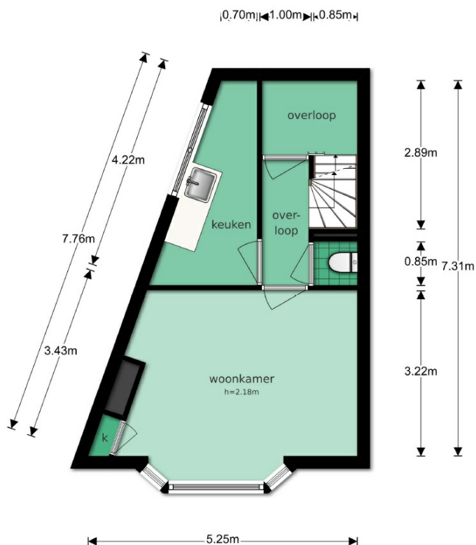
Eerste Verdieping
